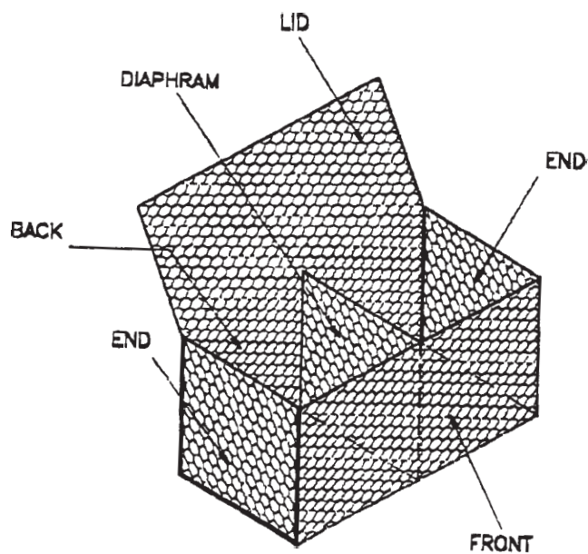
FIG. 1 Gabion
